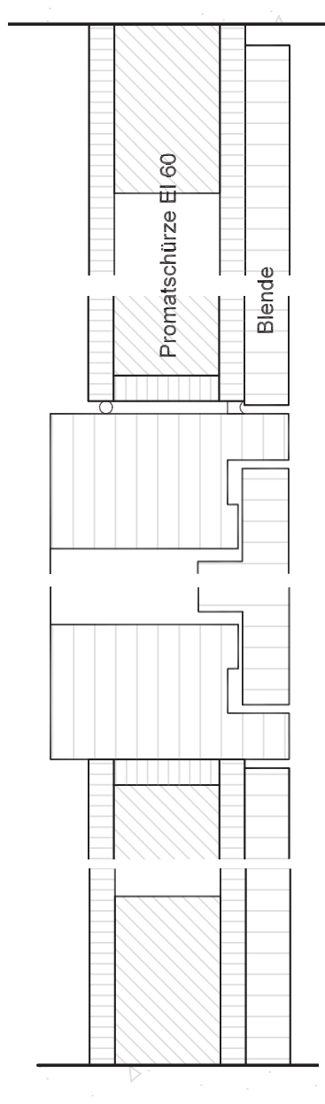
Anschluss Detail 1 vertikal
